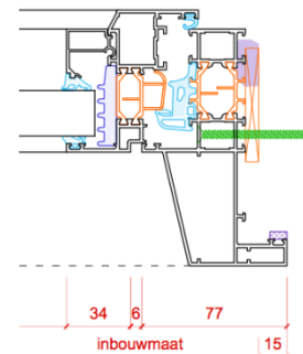
Draaikiepraam
