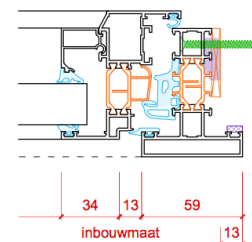
Draaikiepraam
